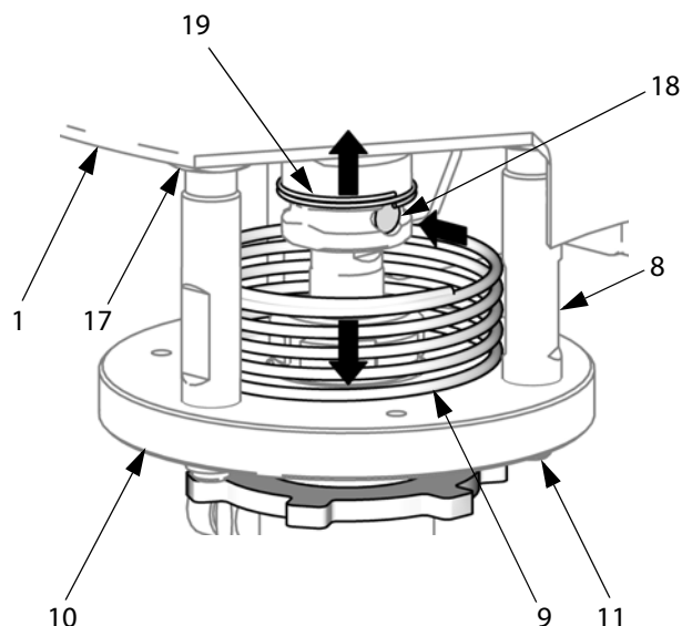
Рис. 12. Отсоединение пневмодвигателя
