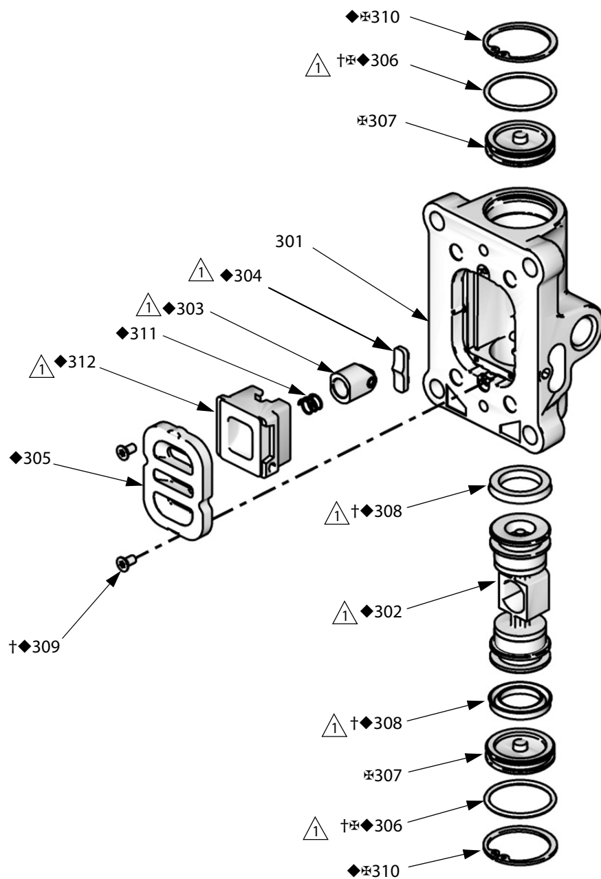
Рис. 9. Сборка воздушного клапана
