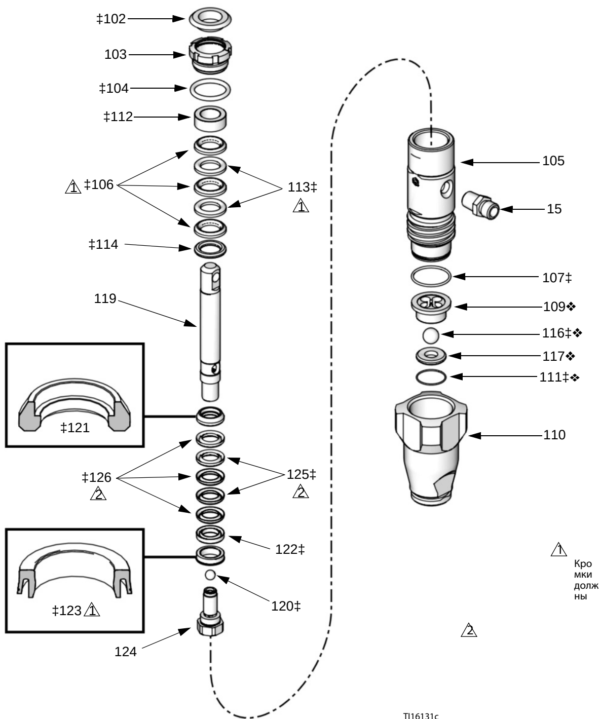
Рис. 7. Поршневой насос
