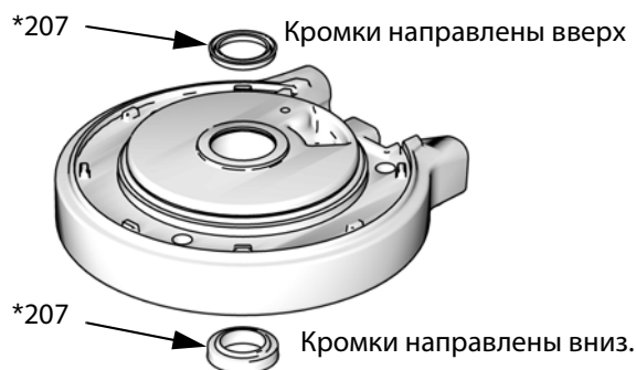
Рис. 13. Установка П-образных уплотнений пневмодвигателя
