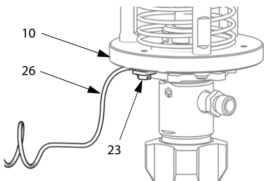
Рис. 1. Провод заземления
